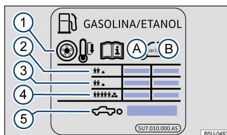
Fig. 162 Etiqueta con las presiones de los neumáticos
