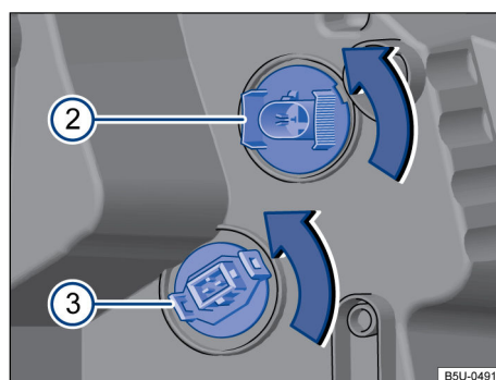
Fig. 136 En el vano motor: vista trasera del faro delantero ② luces diurnas / luz de posición y ③ indicadores de dirección.
