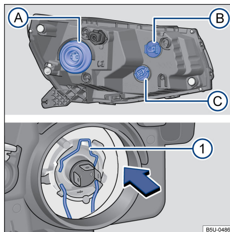
Fig. 135 En el vano motor: vista trasera del faro delantero con cubierta de goma (lado izquierdo de la ilustración) - ① luz de cruce / luz de carretera ② luz de conducción / luz de posición y ③ indicadores de dirección. Vista trasera del farol delantero sin cubierta de goma (lado derecho de la ilustración): ① resorte de bloqueo de la lámpara incandescente del farol bajo/farol alto.
