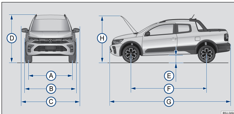
Fig. 179 Dimensiones.
