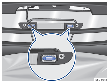
Fig. 142 Linterna de freno elevada: remover la lámpara incandescente de iluminación del compartimento de carga.
